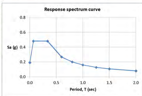
รูปที่ 7 สเปกตรัมผลตอบสนองสำหรับหลุมเจาะ BH-5
