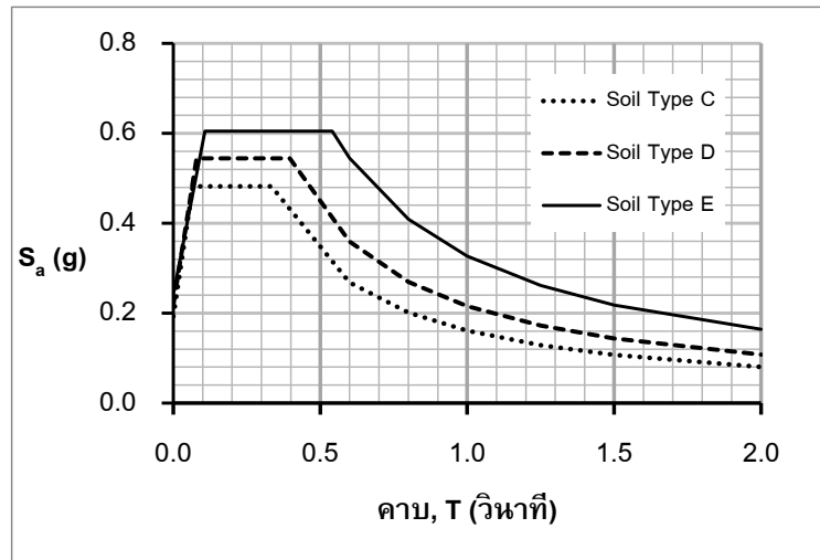
รูปที่ 8 สเปกตรัมผลตอบสนองสำหรับอำเภอเมือง จังหวัดพะเยา จากข้อมูลผลเจาะสำรวจดินทั้ง 35 หลุม
